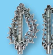
8 TÊTES À CHAÎNES Pour nettoyer des canalisations en acier ou en fonte. Les chaînes dentelées sont utilisées pour le nettoyage des canalisations très engorgées.
